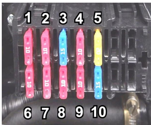
Rys. 5.4.2. Rozmieszczenia bezpieczników w skrzynce
