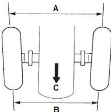
Rys. 5.7.2. Ustawianie zbieżności kół przedniej osi.
