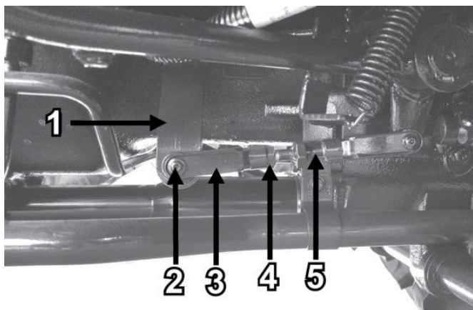
Rys. 5.8. Regulacja skoku pedału sprzęgła
