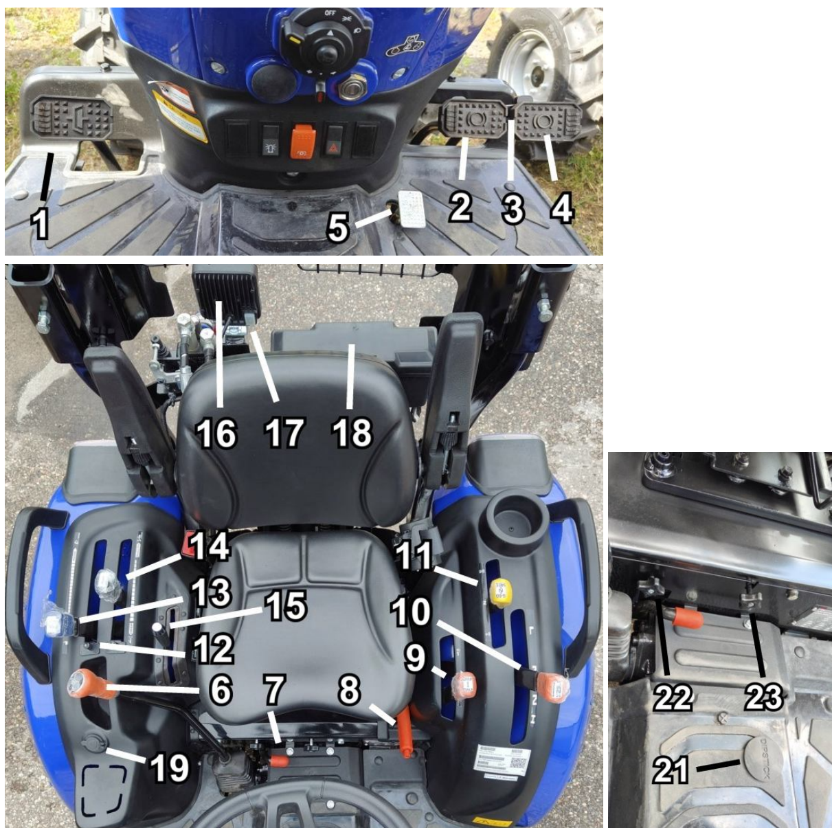
Rys. 3.2. Dźwignie sterowania ciągnikiem - opis w tekście
